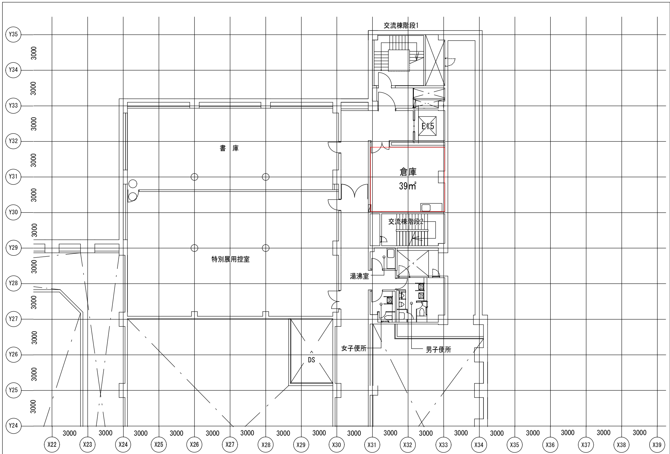
東京都美術館 B3F : ミュージアムショップ倉庫 平面図
